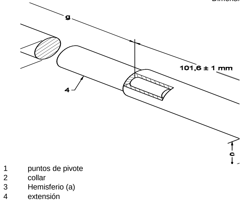
Figura 17. Sonda de accesibilidad
